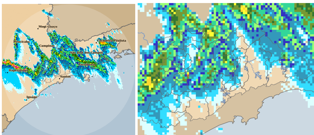
Figura 4: Acumulado no Período: 28/01/2024 08:30 a 28/01/2024 21:50 GMT
