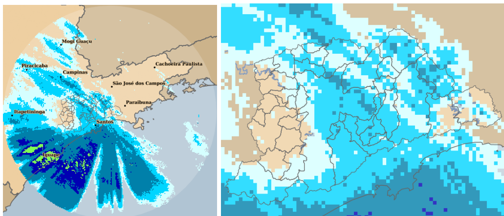
Figura 4: Acumulado no Período: 09/09/2023 04:00 a 10/09/2023 12:30 GMT
