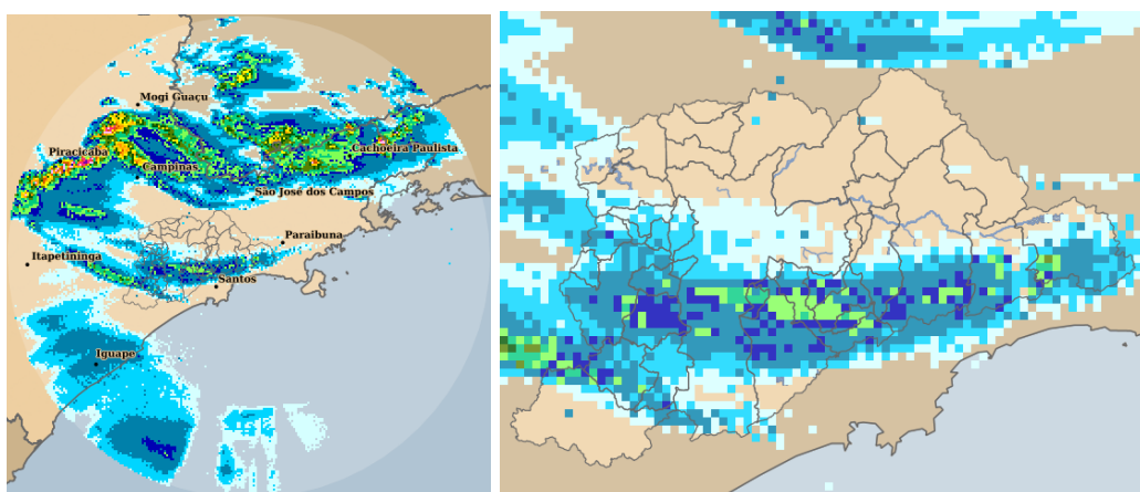
Figura 4: Acumulado no Período: 12/08/2023 16:10 a 13/08/2023 02:05 GMT
