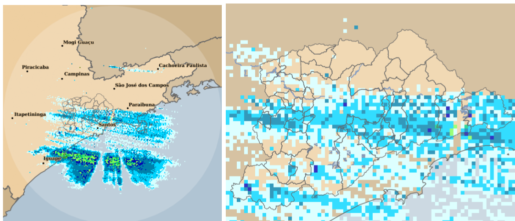
Figura 4: Acumulado no Período: 17/07/2023 03:00 a 17/07/2023 14:00 GMT
