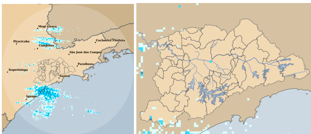
Figura 4: Acumulado no Período: 16/07/2023 10:30 a 17/07/2023 00:35 GMT
