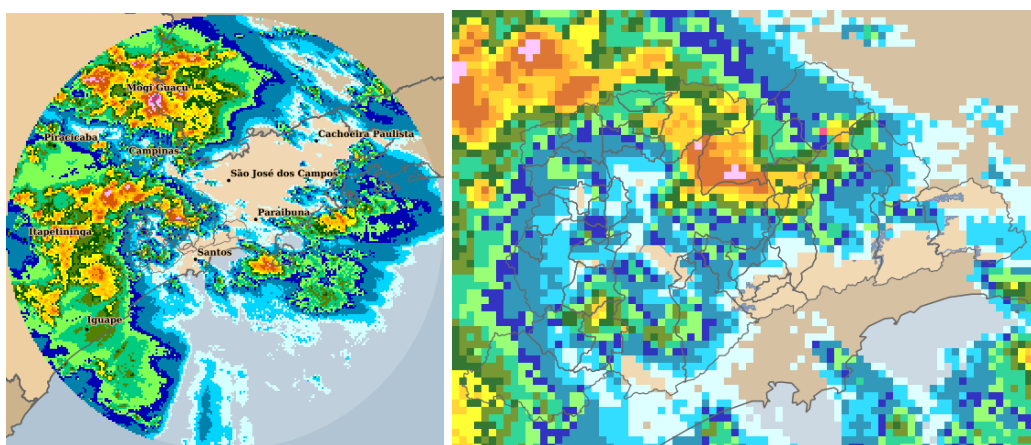
Figura 4: Acumulado no Período: 29/03/2023 15:30 a 30/03/2023 12:30 GMT
