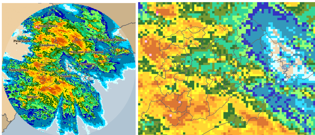
Figura 4: Acumulado no Período: 05/03/2023 19:20 a 06/03/2023 09:30 GMT
