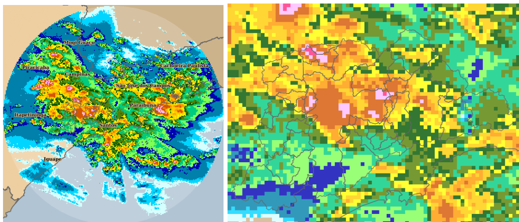
Figura 4: Acumulado no Período: 07/02/2023 12:00 a 08/02/2023 06:20 GMT
