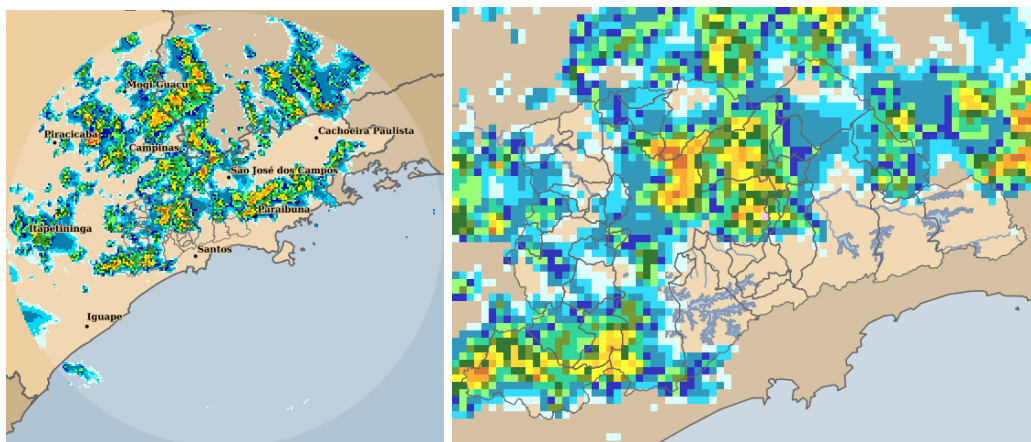
Figura 4: Acumulado no Período: 11/10/2017 14:00 a 12/10/2017 02:00 GMT
