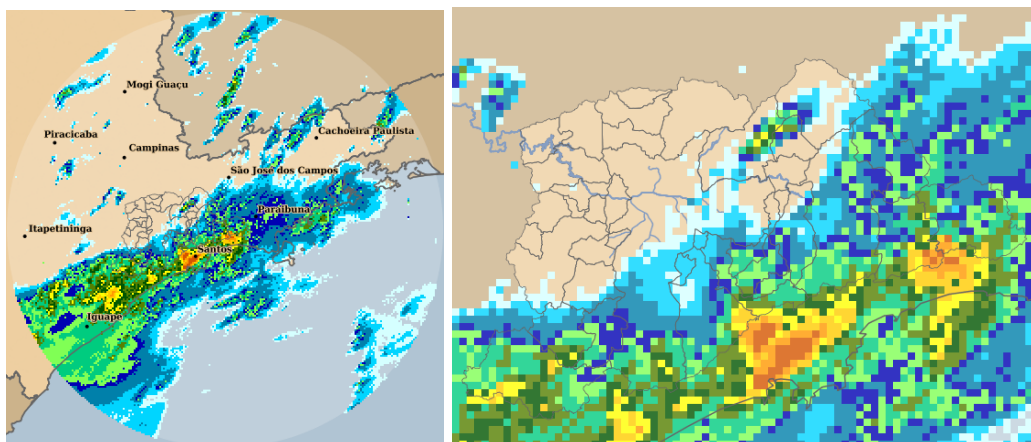
Figura 4: Acumulado no Período: 11/04/2017 16:54 a 12/04/2017 14:44 GMT
