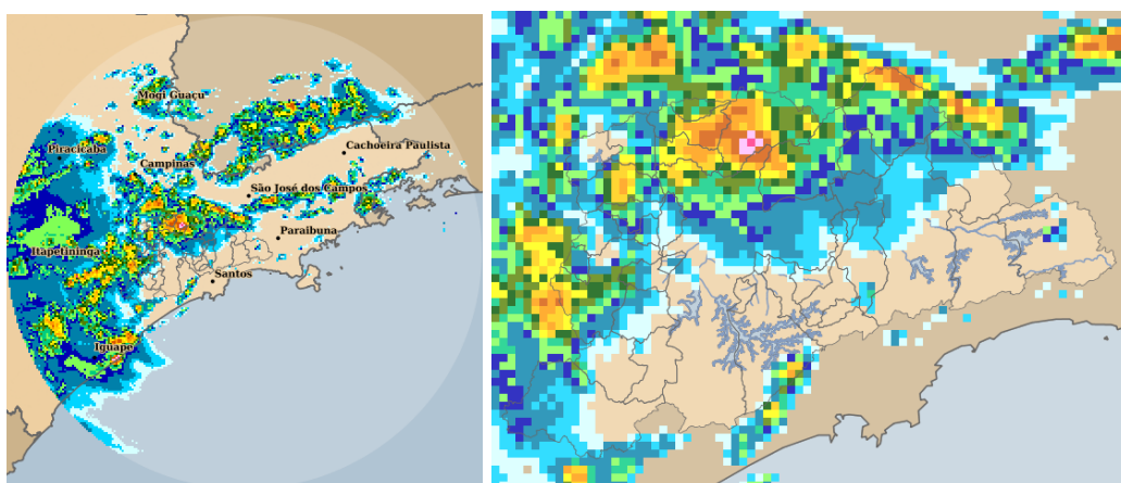
Figura 4: Acumulado no Período: 30/01/2017 10:00 a 31/01/2017 01:59 GMT
