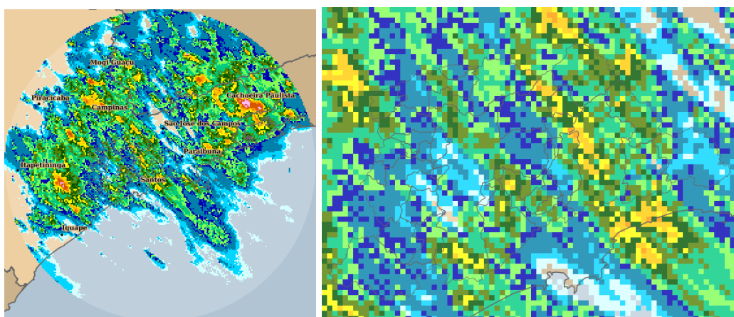
Figura 4: Acumulado no Período: 24/01/2017 14:14 a 25/01/2017 07:59 GMT
