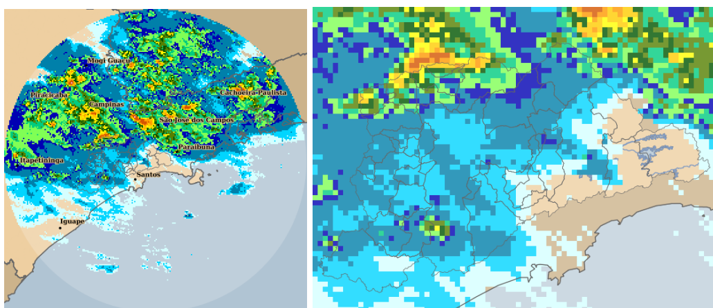
Figura 4: Acumulado no Período: 09/12/2016 14:00 a 10/12/2016 11:00 GMT
