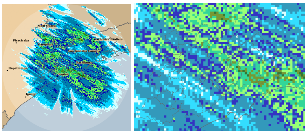
Figura 4: Acumulado no Período: 27/10/2016 11:45 a 28/10/2016 00:55 GMT
