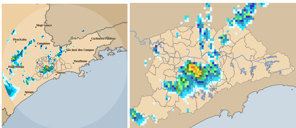
Figura 4: Acumulado no Período: 09/03/2016 17:45 a 09/03/2016 22:35 GMT
