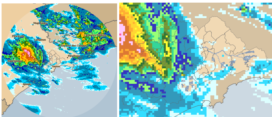
Figura 4: Acumulado no Período: 25/02/2016 12:50 a 26/02/2016 09:50 GMT
