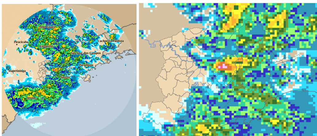
Figura 4: Acumulado no Período: 25/01/2016 14:00 a 26/01/2016 03:45 GMT
